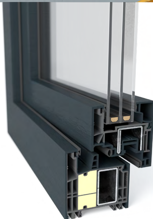
GEALAN-KONTUR® okvir s 2 velike IKD® komore
